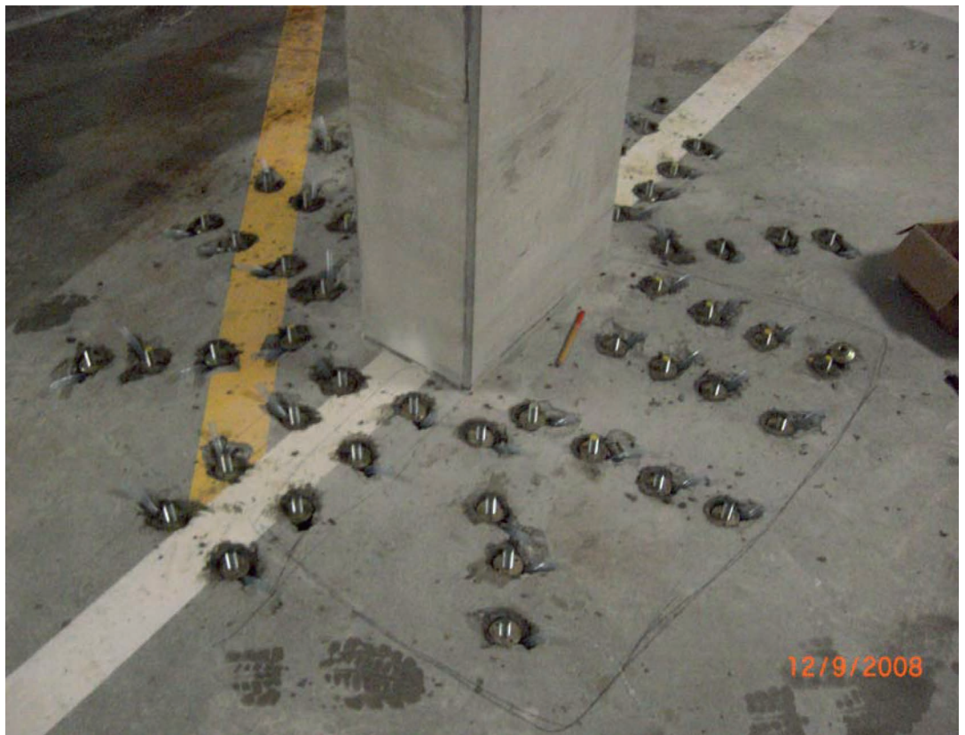
Vergiessen der ancoSAN® mit spez. Fließmörtel
