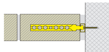
XLS aufgedübelt rail fixé avec cheville
