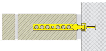
ATA einbetoniert embétonné
