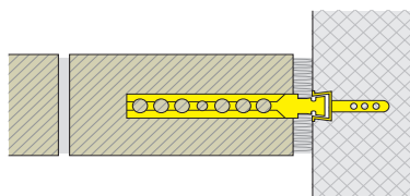
XMS einbetoniert rail embétonné
