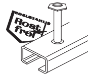
Ankerschienen und Hammerkopfschraube Rail d'ancrage et Boulon à tête marteau
