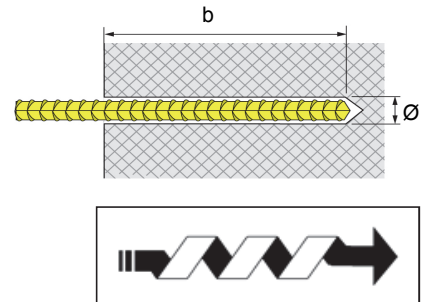
TB-Verankerungsseisen Fer d'armature TB
