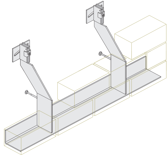
Winkelkonsolen AKO
