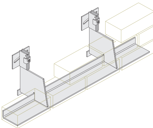
Abfangkonsolen AKN
