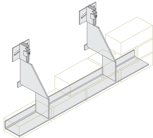
Winkelkonsolen AKO
