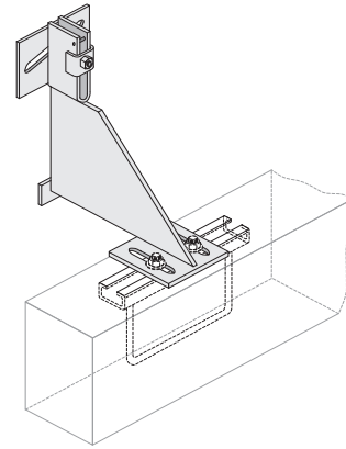
Winkelkonsolen AKM
