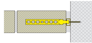
XLS aufgedübelt rail fixé avec cheville
