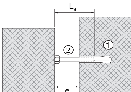
vorfabriziertes Element élément préfabriqué
