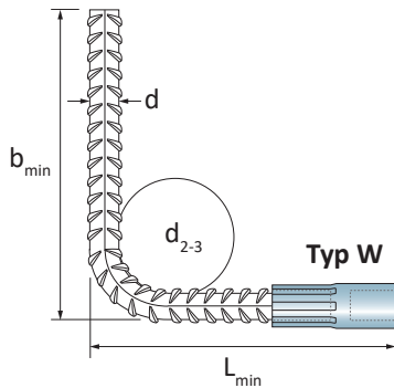
BARON®-C Muffenstab gebogen (Typ W)
