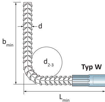
BARON®-C Muffenstab gebogen (Typ W)
