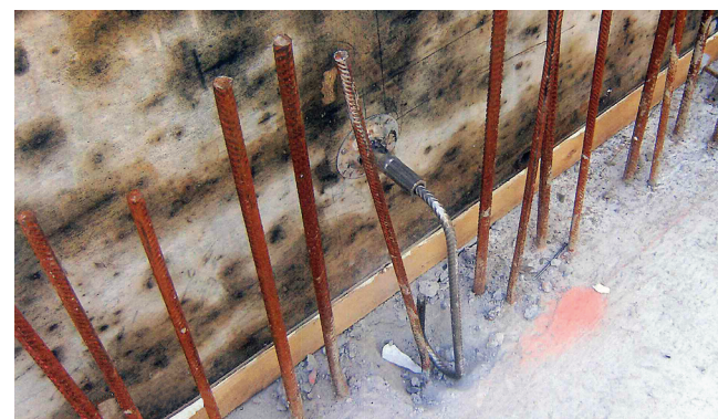
Zuganker im Einsatz auf der Baustelle. Ancre de traction en utilisation sur le chantier.
