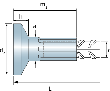
Typ / type E (BARON®-C)
