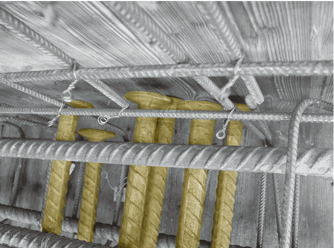
Einspannung der Fahrbahnplatte in einer Wand im Parkhaus. Encastrement d'une dalle en porte-à-faux pour une rampe hélicoïdale de parking.
