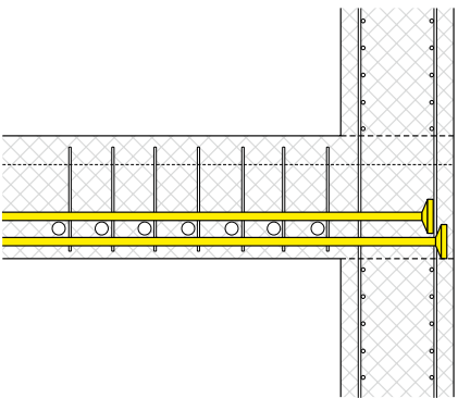
Einspannung der Fahrbahnplatte in einer Wand im Parkhaus. Encastrement d'une dalle en porte-à-faux pour une rampe hélicoïdale de parking.
