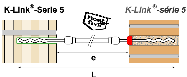
Sanierungsanker (inkl. eine Siebhülse) Ancre d'assainissement (1 tamis incl.)
