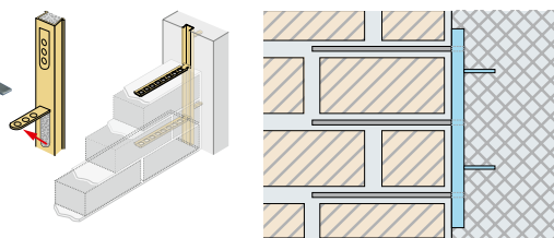
Rails de raccordement pour murs
