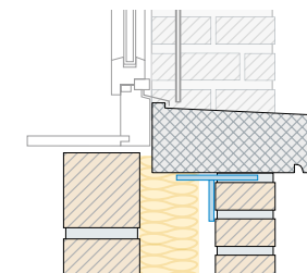
Appui pour tablette de fenêtre FBK
