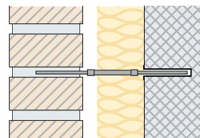
Ancre à double articulation KE
