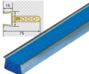
MURINOX®- Maueranschlussschiene
