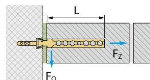
Wandanschluss Liaison de murs
