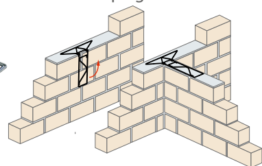
Epingle de liaison KLP
