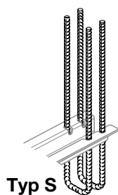
Typ S horizontal
