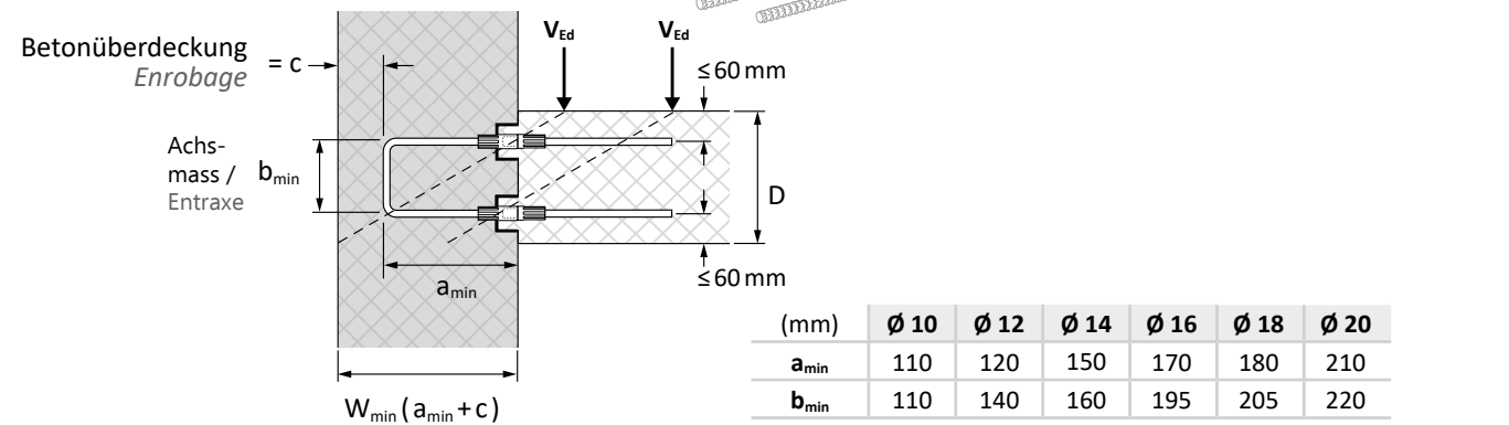
Typ BU: Verbindung (Wand-Decke)
