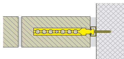
Maueranschluss mit ML-Anker (S.90) Liaison de murs avec ancre ML (p.90)
